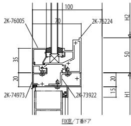
FIX窓/丁番ドア
