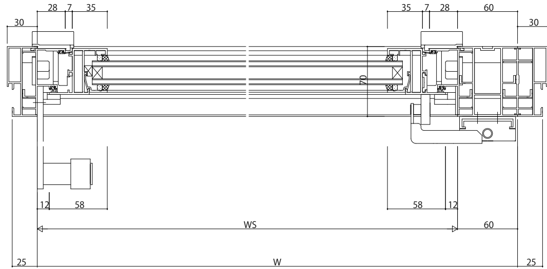
B-B断面
