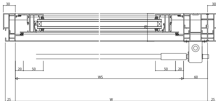
A-A断面
