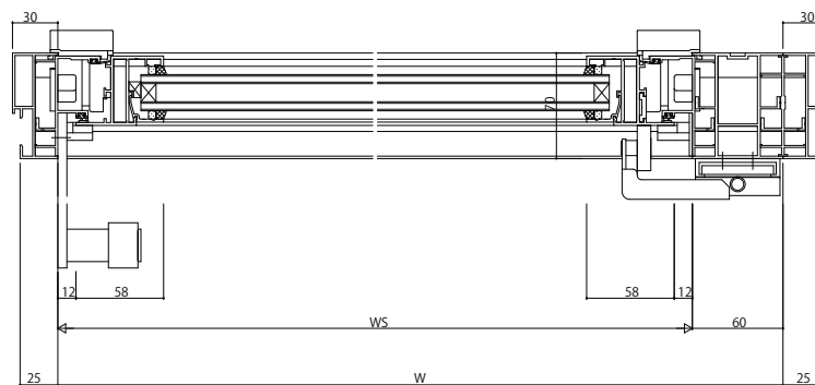
B-B断面
