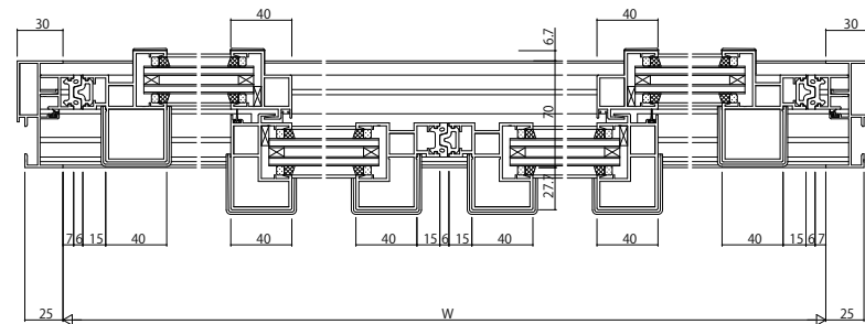
4枚建Cタイプの場合
