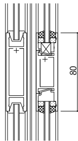
中棧 (80見付)
