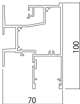
■ F I X ( 1 8 ・ 2 8 mm ) / 片引き [ 2 K - 8 4 4 2 3 ]
