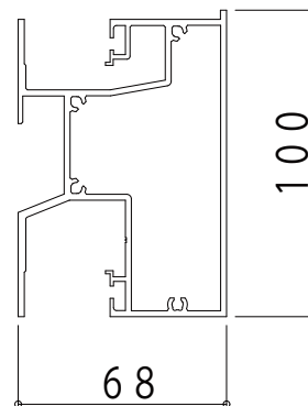
■ F I X / F I X ( 1 8 ・ 2 8 mm ) [ 2 K - 9 5 8 3 0 ]
