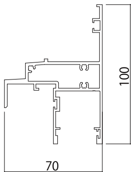
■ 外倒し・突出し【排煙窓・隠ぺい】/ 片引き [ 2 K - 8 4 4 2 4 ]
