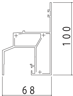
■ 外倒し・突出し【排煙窓・隠ぺい】/ F I X ( 3 8 mm ) ■ F I X ( 1 8 ・ 2 8 mm ) / 可動 [ 2 K - 8 4 4 8 7 ]
