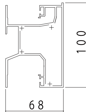
■ F I X / F I X ( 1 8 ・ 3 8 mm ) [ 2 K - 8 4 4 8 4 ]
