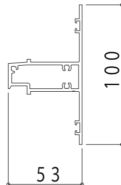
■ 可動 / 可動 [ 2 K - 9 5 8 3 3 ]
