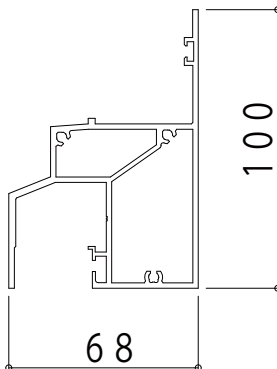
■ 可動 / F I X ( 1 8 ・ 2 8 mm ) [ 2 K - 9 5 8 3 2 ]
