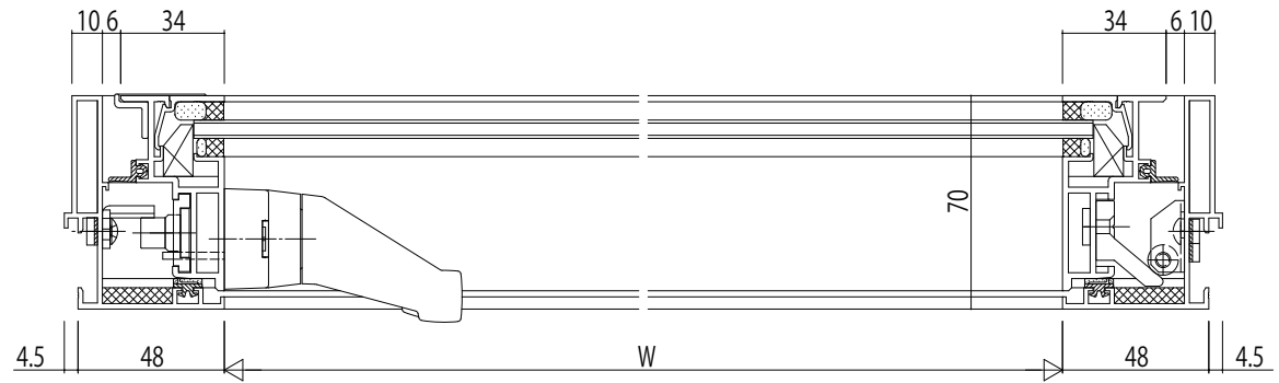
たて骨部(たてすべり出し+FIX)
