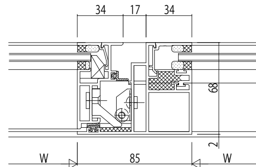
たて骨部(たてすべり出し+FIX)
