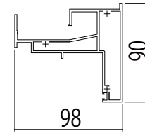
●FIX(38・48mm)/大型たてすべり出し [2K-75387]
