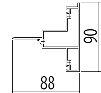
●可動/たてすべり出し [2K-75386]
