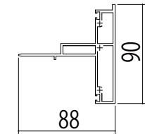
●可動/大型たてすべり出し [2K-75389]
