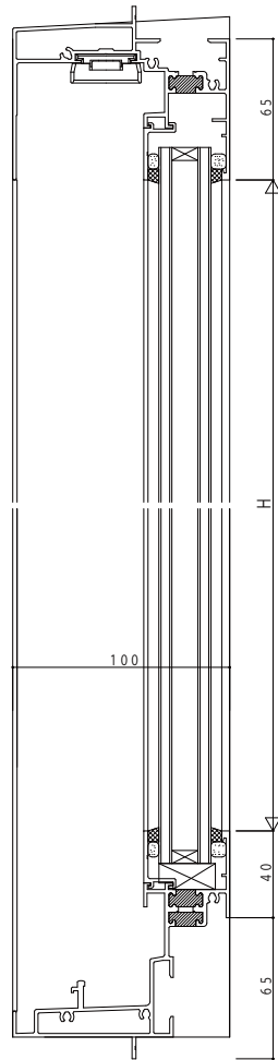
はめ殺し部
