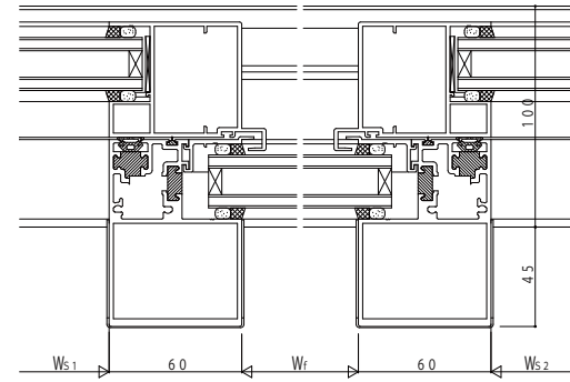
煙返し無
