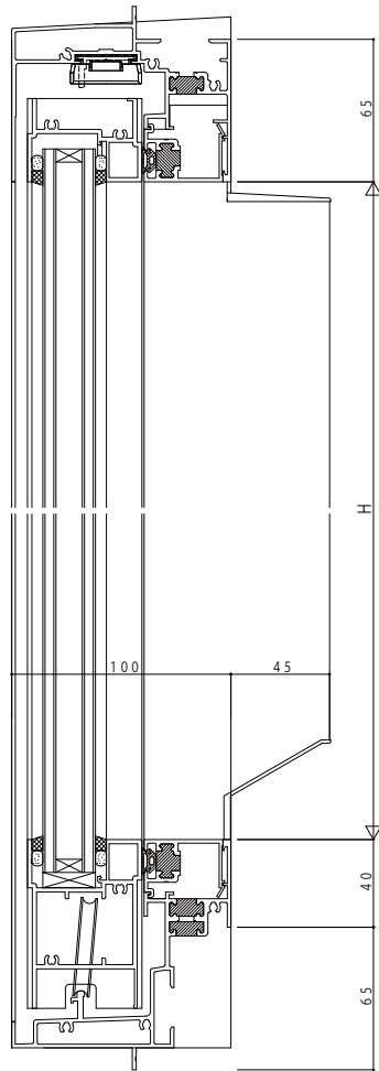
障子部
