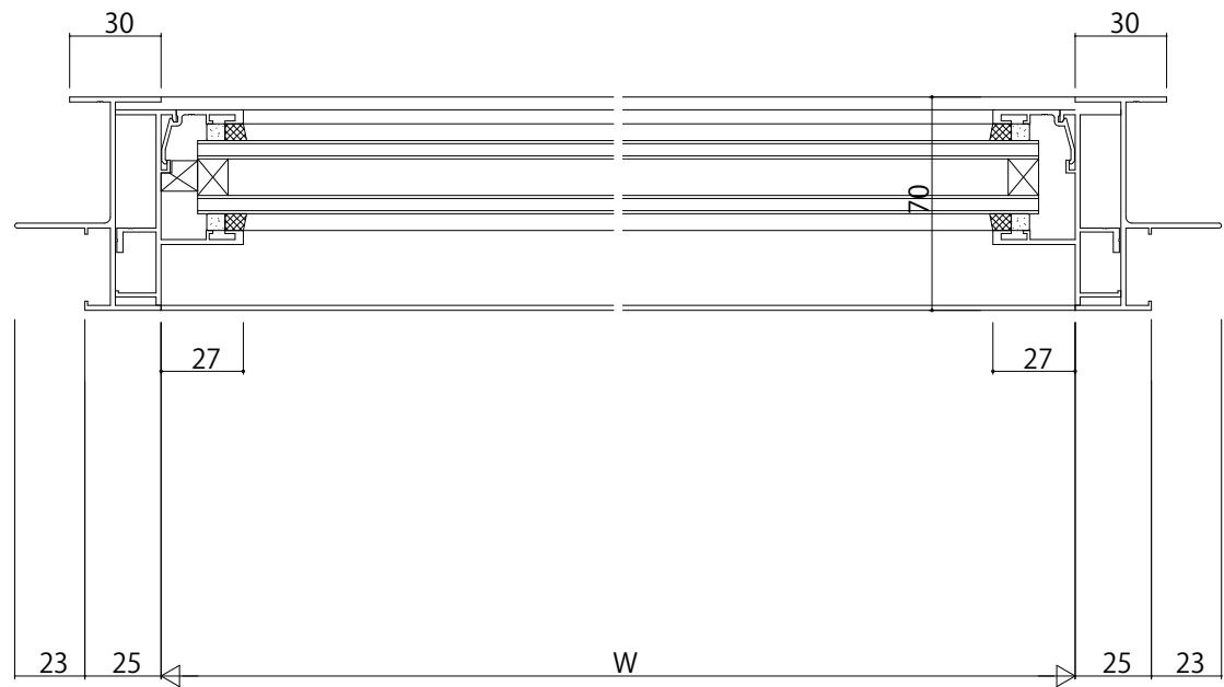
たて中骨
