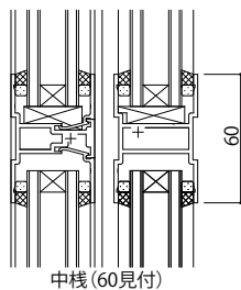
中棧 (60見付)
