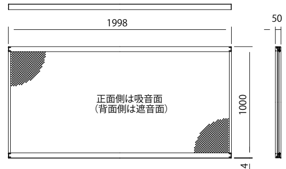
パネル (吸音タイプ H1m) 詳細図 (1/25)
