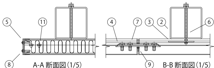
A-A 断面図 (1/5)
