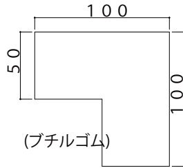
鉄骨枠用2K-24405
