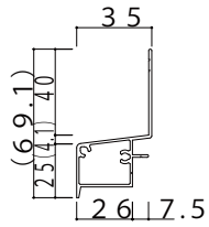
上見切縁K-88290
