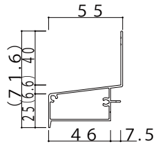
上見切縁K-88293
