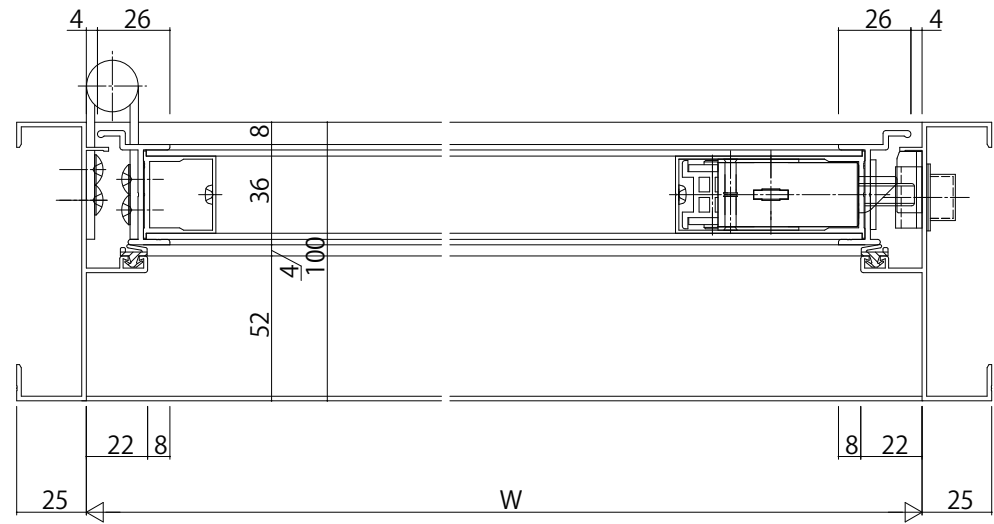
両開き召合せかまち部
