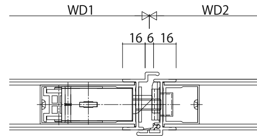
両開き召合せかまち部
