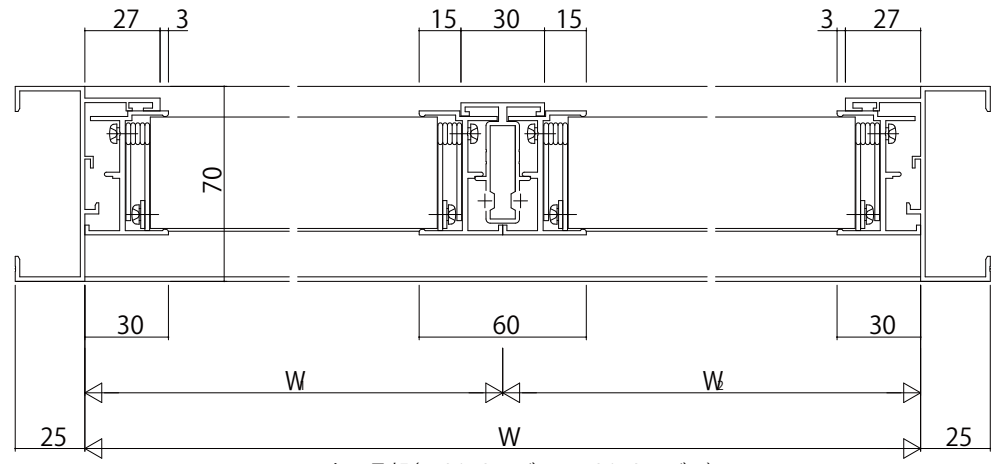
たて骨部(アルミルーバー+アルミルーバー)
