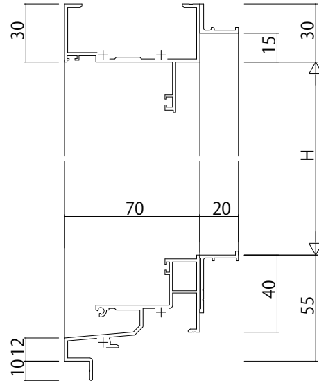
RC枠 アンゲル付
