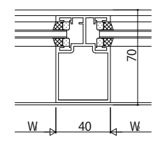
たて骨 (40見付)
