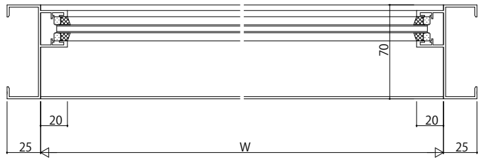
たて骨
