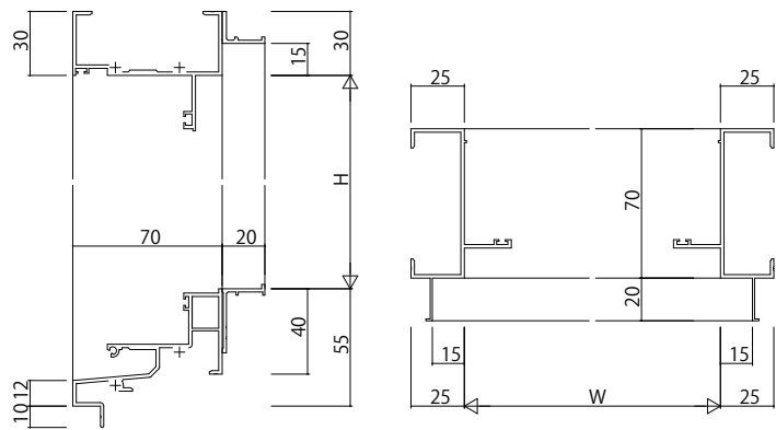
RC枠 アンゲル付
