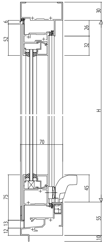
カムラッチハンドル
