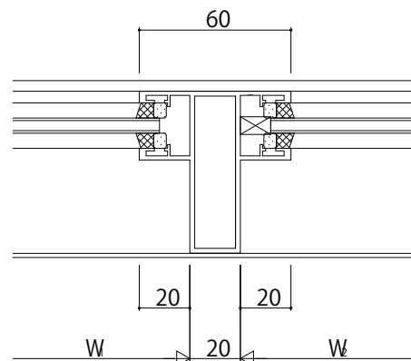
たて中骨
