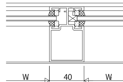
たて中骨(40見付)
