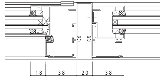
たて骨部(オーニング+FiX)
