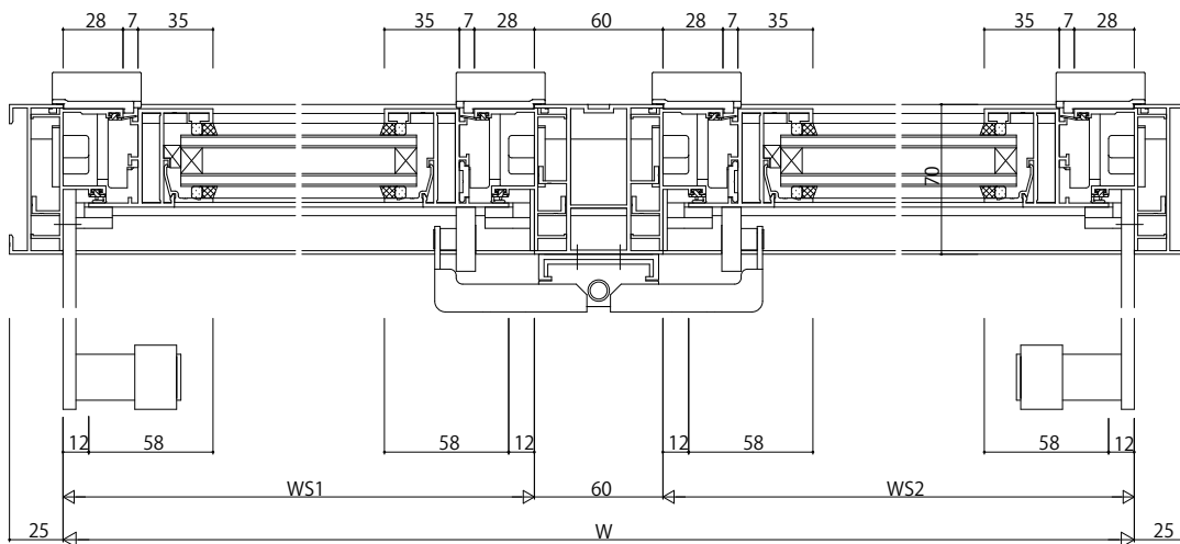
A-A断面
