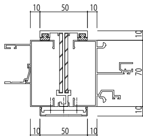
●A方立
