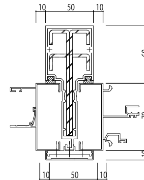
●D方立
