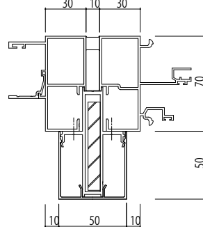
●B方立
