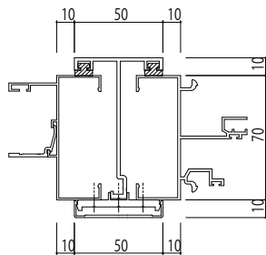
●SA方立
