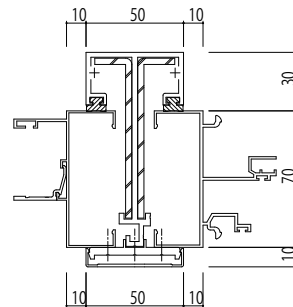
●C方立
