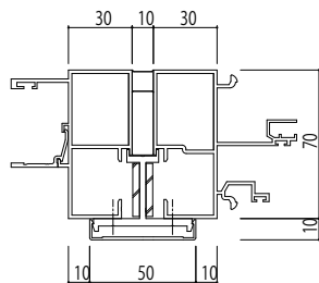
●A方立
