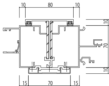
●A方立
