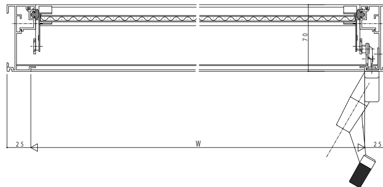
たて骨部(ガラスルーバー+FIX)
