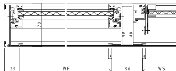
たて骨部(ガラスルーバー+FIX)
