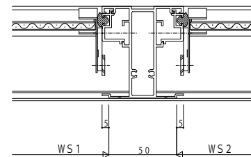
たて骨部(ガラスルーバー+ガラスルーバー)
