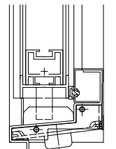
下枠ステンレス
