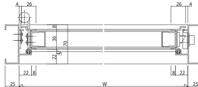
両開き突合せかまち部
