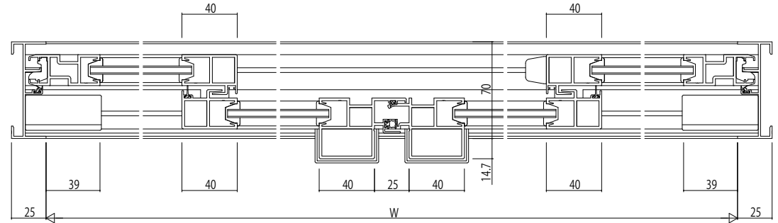
4枚建 Aタイプの場合
