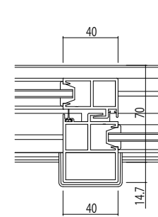
4枚建 Bタイプ召合せかまちの場合
