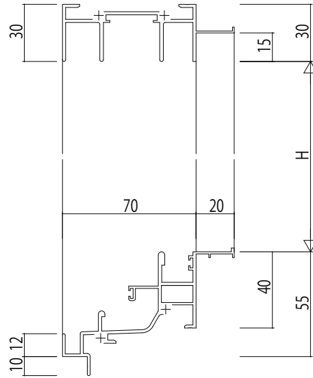
RC枠 アングル付
