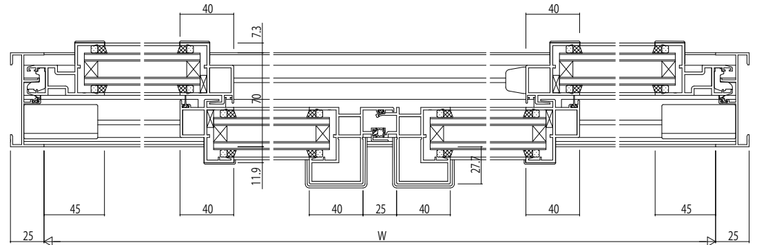
4枚建 Aタイプの場合
