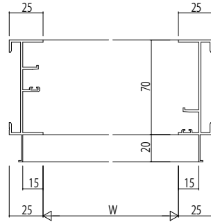
RC枠 アングル付2枚建
