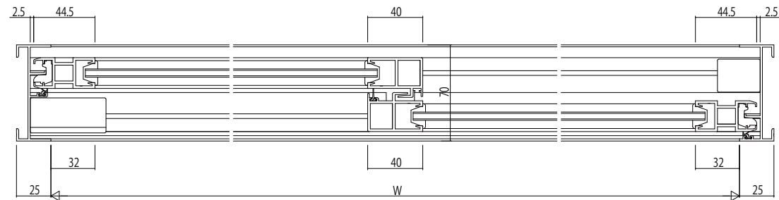
4枚建 Aタイプの場合
