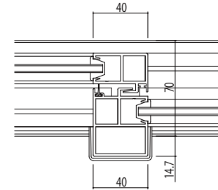
Bタイプ召合せかまち部
