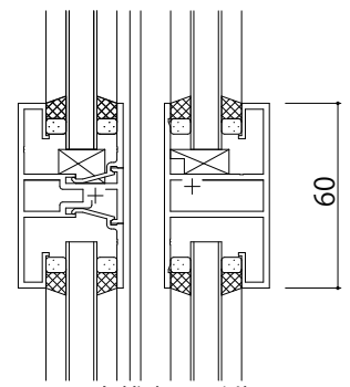
中棧(60見付)
