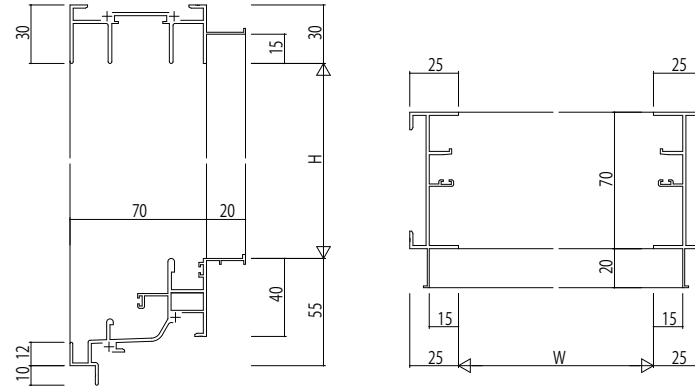
RC枠 アンゲル付
