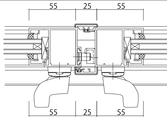
両開き召合せ部(グレモン)
