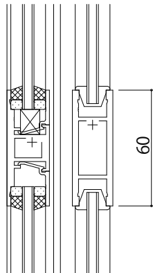
中棧 (60見付)
