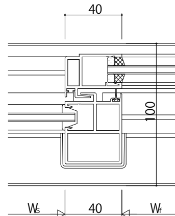
Bタイプ召合せかまち
