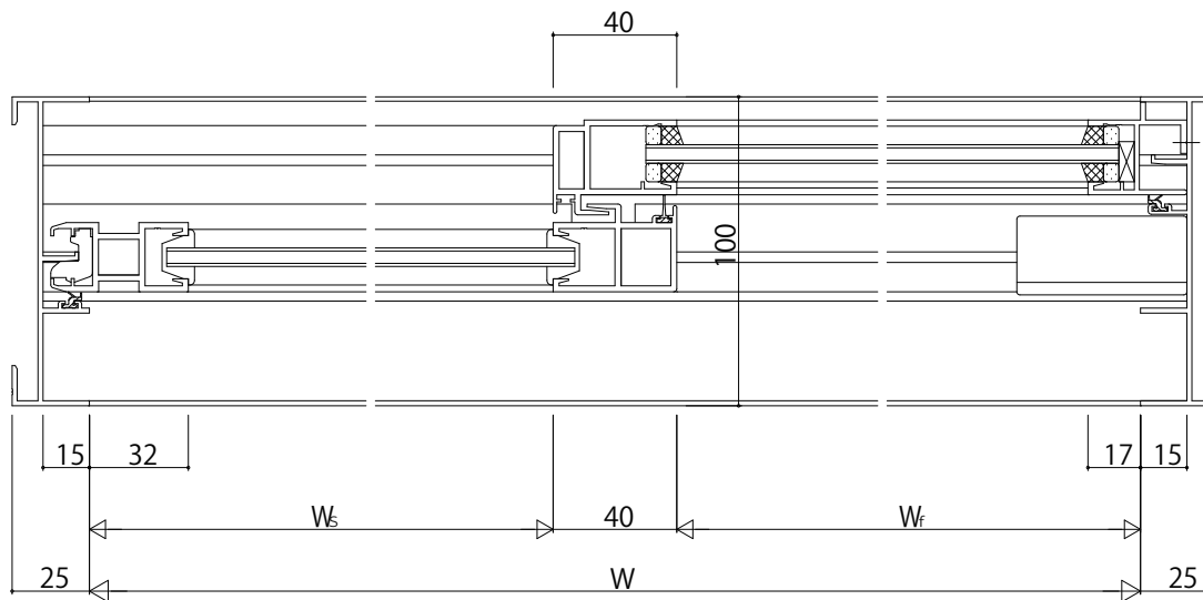
Aタイプ召合せかまち
