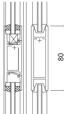
中棧 (80見付)
