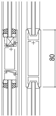
中棧(80見付)
