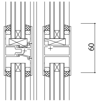
中棧(60見付)
