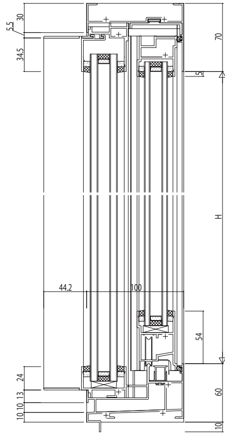
FIX部42mm溝幅
