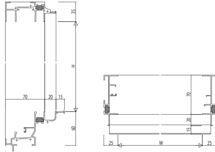
(2)引違い ■RC枠 ●結露受アングル付
