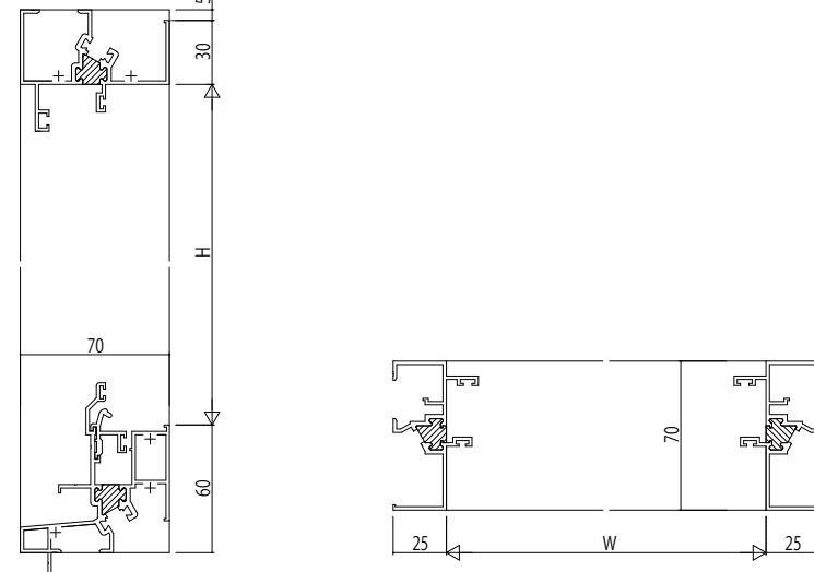
(4)内倒し窓 ■RC枠 ●アングルなし
