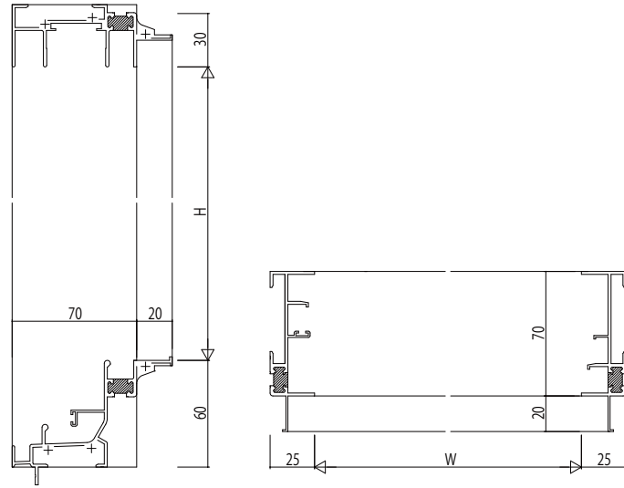
(1)引違い ■RC枠 ●アングル付
