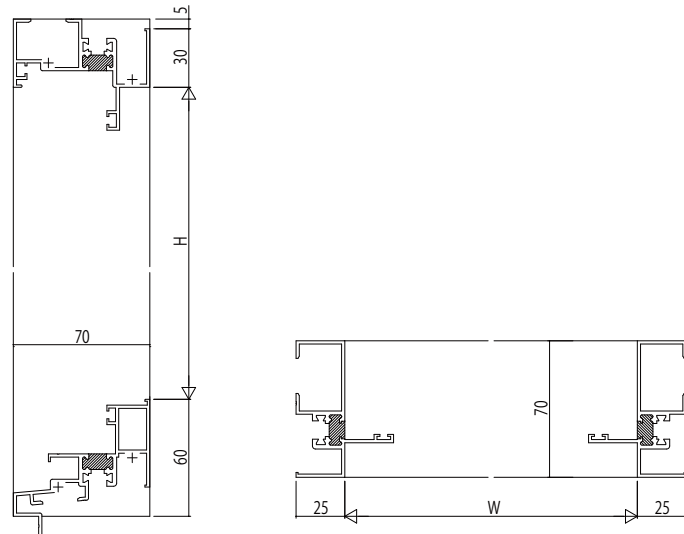
(3)たてすべり出し窓 ■RC枠 ●アングルなし
