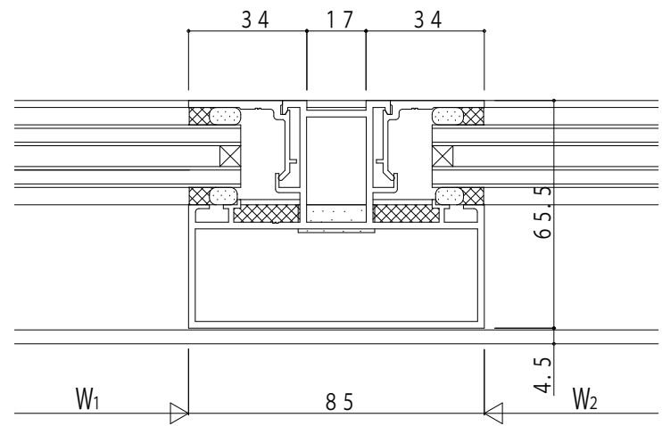
たて骨部(FIX+FIX)
