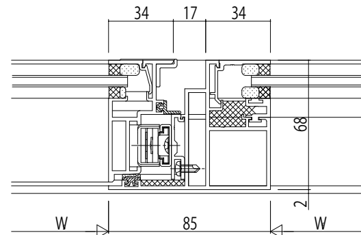
たて骨部(すべり出し+F I X)
