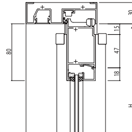
ランマなしの場合
