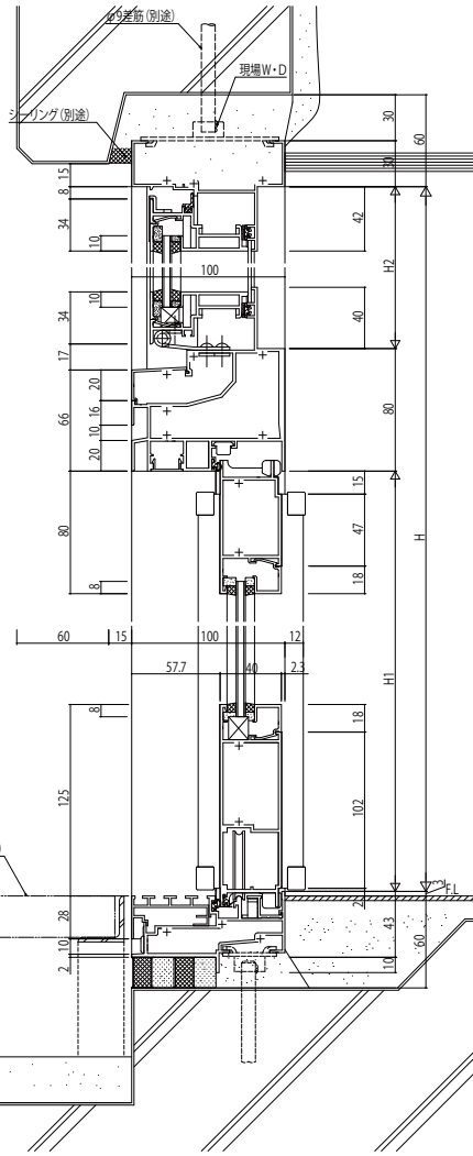
扉部 外倒し窓/片引き戸
