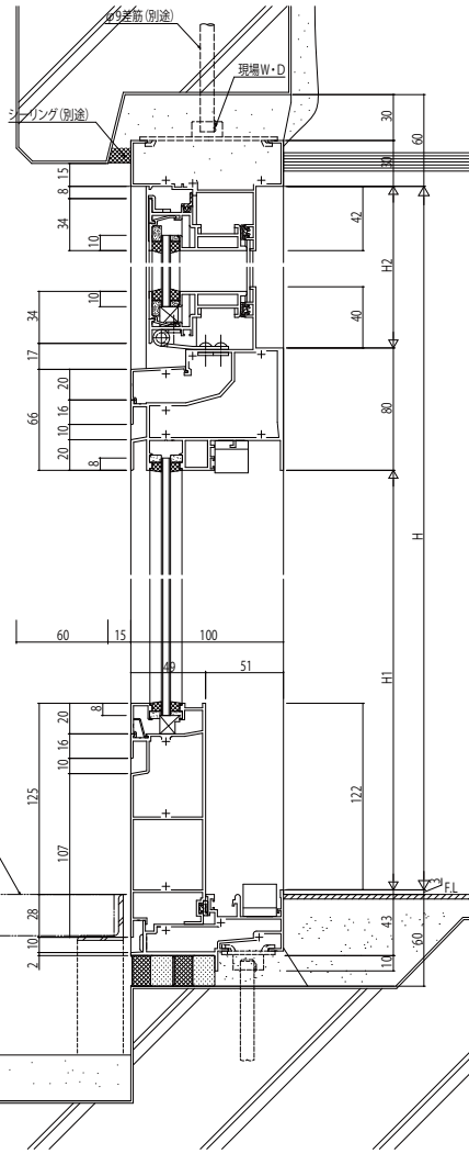
袖FIX部 外倒し窓/片引き戸
