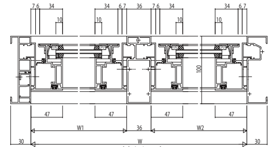
外倒し窓 連窓たて骨連窓
