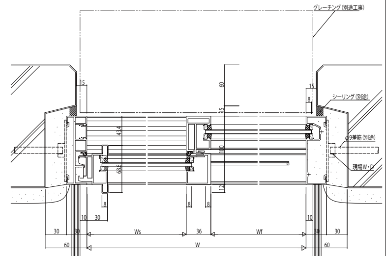
外倒し窓 連窓たて骨連窓
