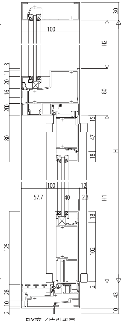
FIX窓/片引き戸
