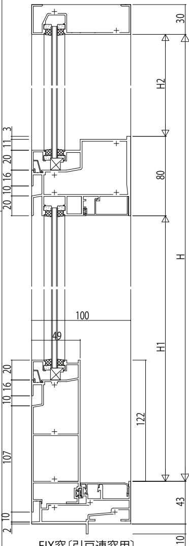
FIX窓(引戸連窓用)
