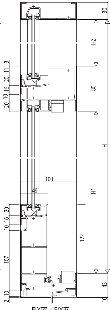
FIX窓/FIX窓
