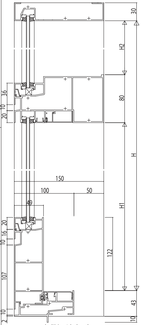
FIX窓(引戸連窓用)
