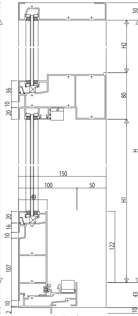
FIX窓/FIX窓
