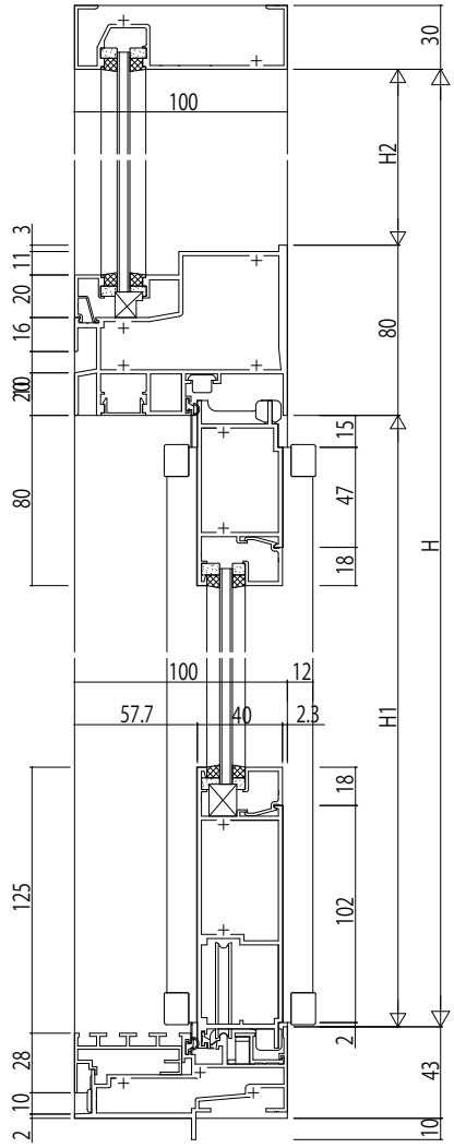
扉部 FIX窓/片引き戸
