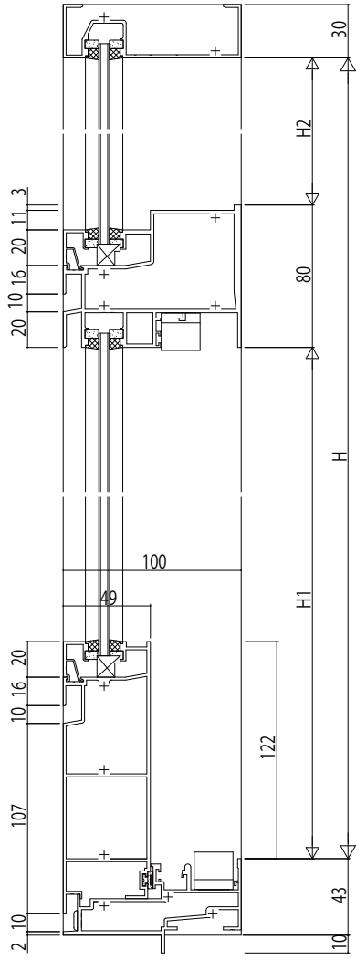
袖FIX部 FIX窓/片引き戸
