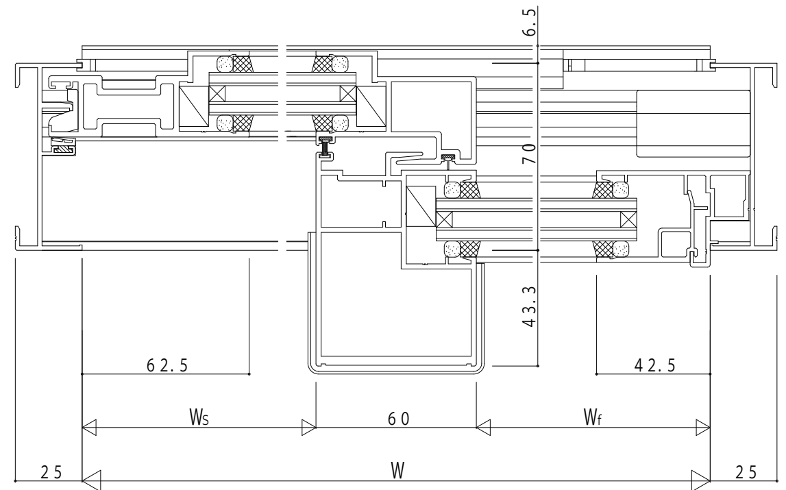
下枠カバー
