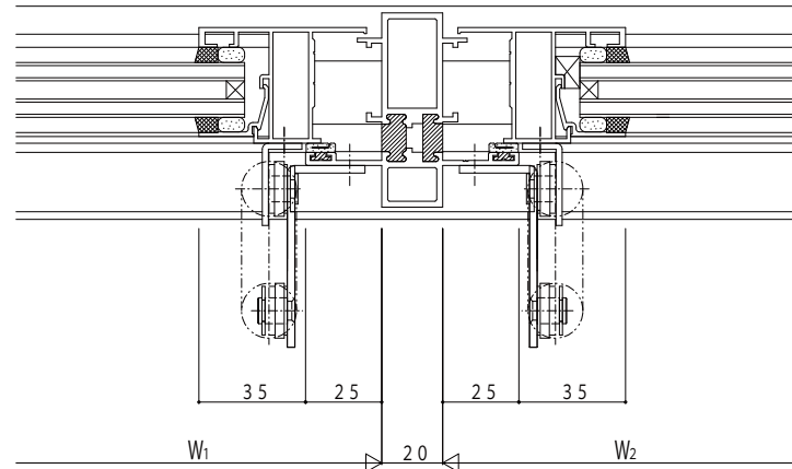
たて骨部(外倒し+外倒し)
