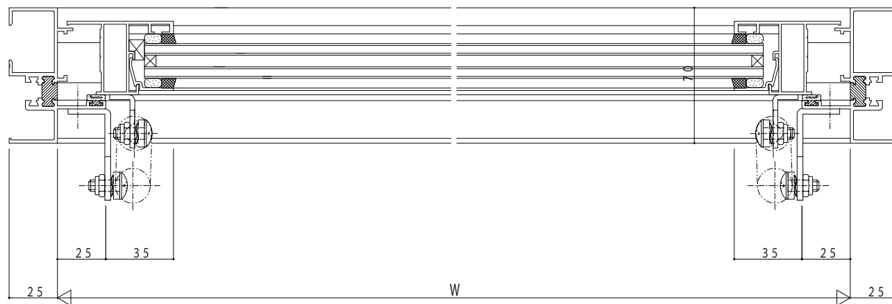
たて骨部 (外倒し+外倒し)
