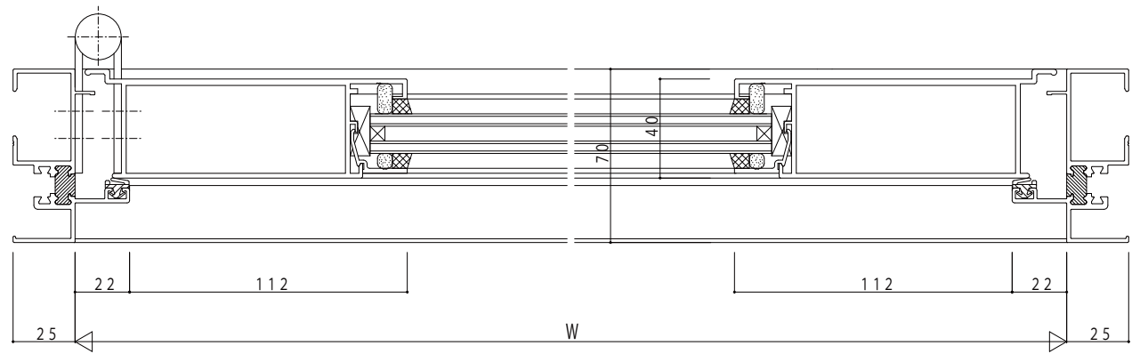
両開き召合せ部
