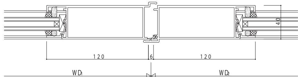
両開き召合せ部
