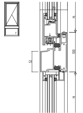
(18) たてすべり出し/FIX
