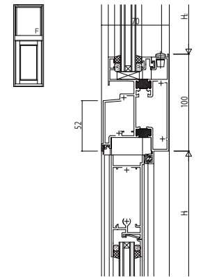
(19) FIX/ドア
