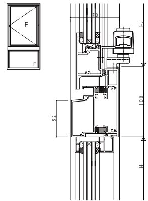
(16) 外開き/FIX
