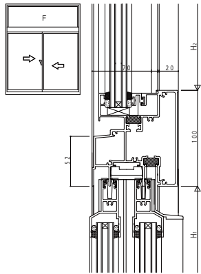
(2) FIX/引違い
