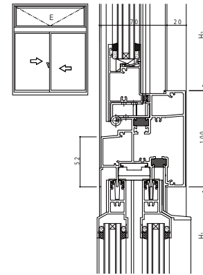
(6) 外倒し(一般・排煙)/引違い
