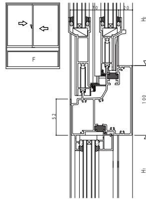
(4) 引違い/FIX
