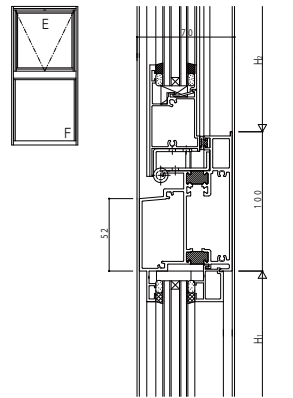
(10) 外倒し(一般・排煙)/FIX
