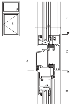
(15) FIX/外開き
