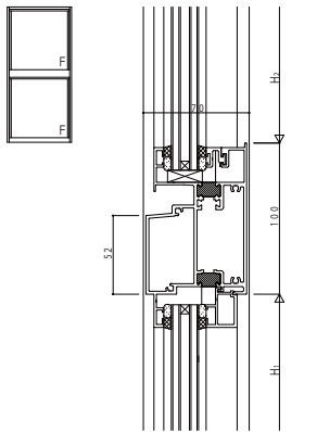
(7) FIX/FIX
