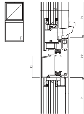
(13) すべり出し/FIX
