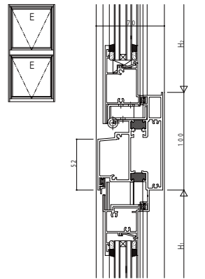
(11) 外倒し(一般)/外倒し(一般)
