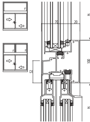
(3) FIX/引違い
