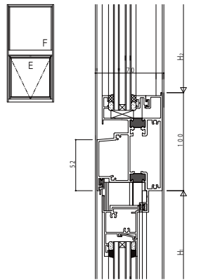
(9) FIX/外倒し(一般・排煙)
