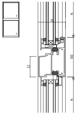
(8) FIX/FIX
