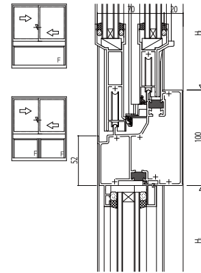
(5) 引違い/FIX
