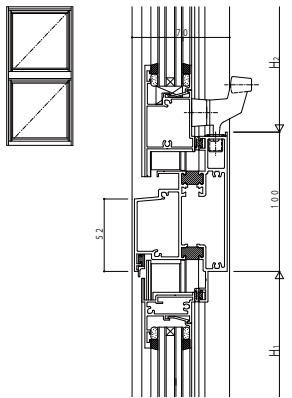
(14) すべり出し/すべり出し
