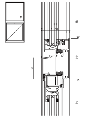
(12) FIX/すべり出し
