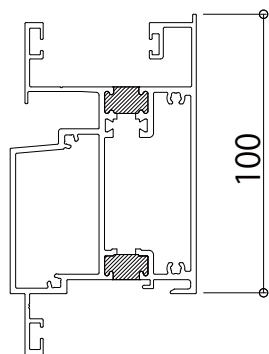
■FIX／FIX
