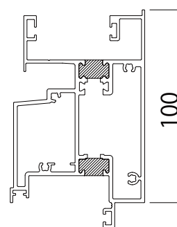
■FIX／ドア
