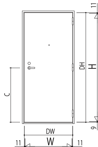
外觀姿図(1/20)
