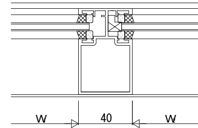
たて中骨 (40見付)
